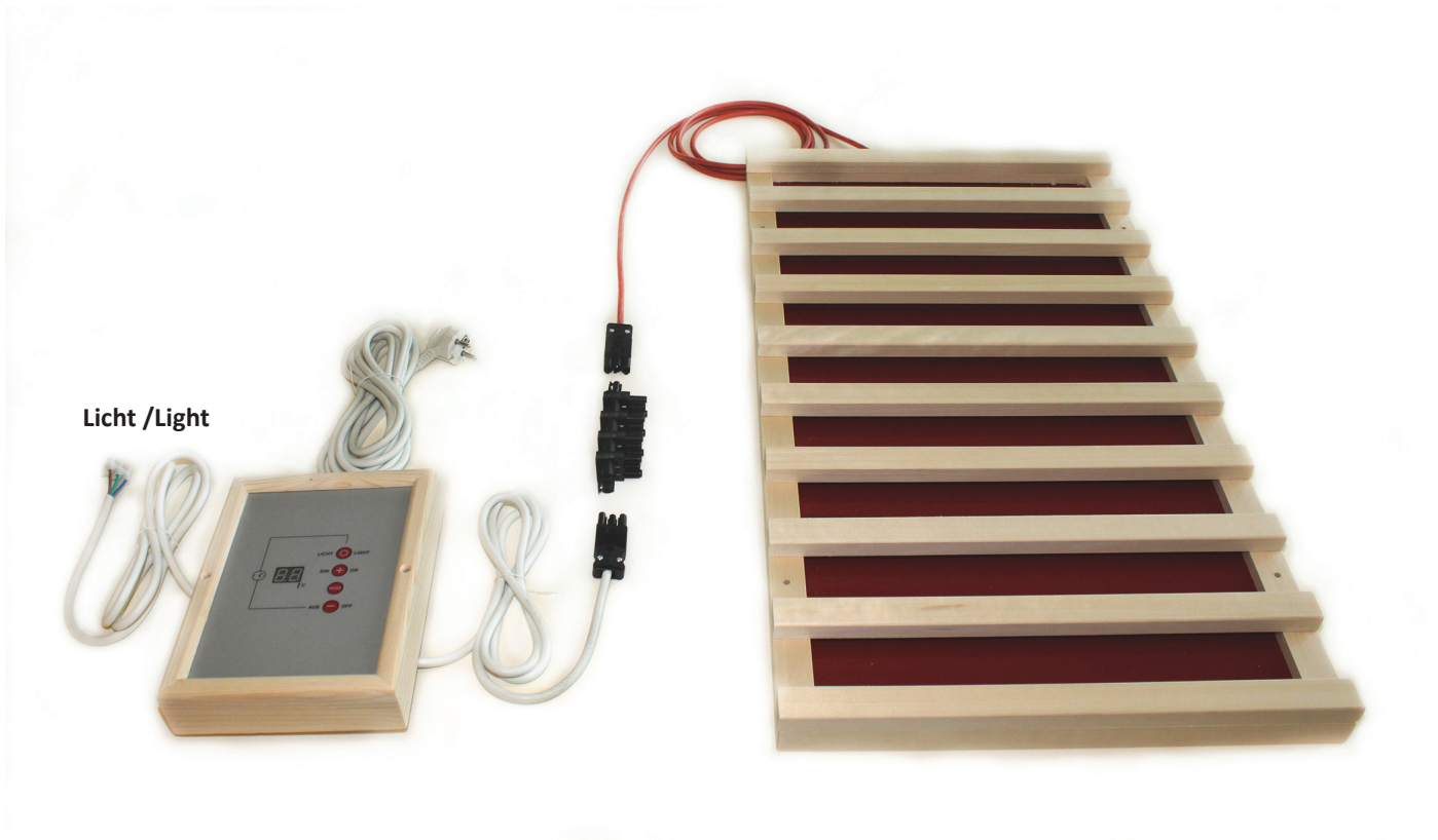
Variante B: Anschluss an Infrarot-Flächenheizung
