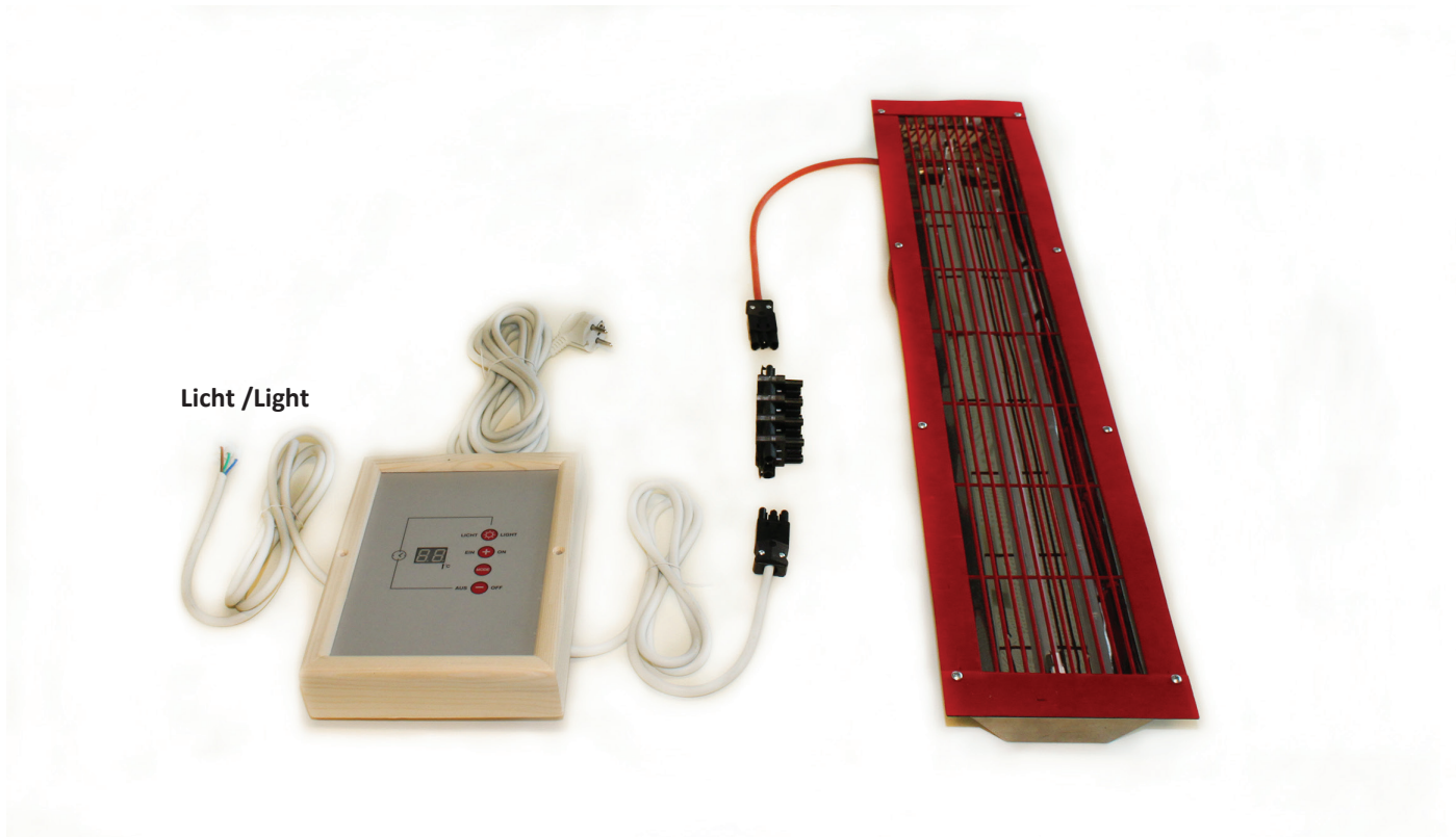
Variante B: Anschluss an Infrarot-Flächenheizung
